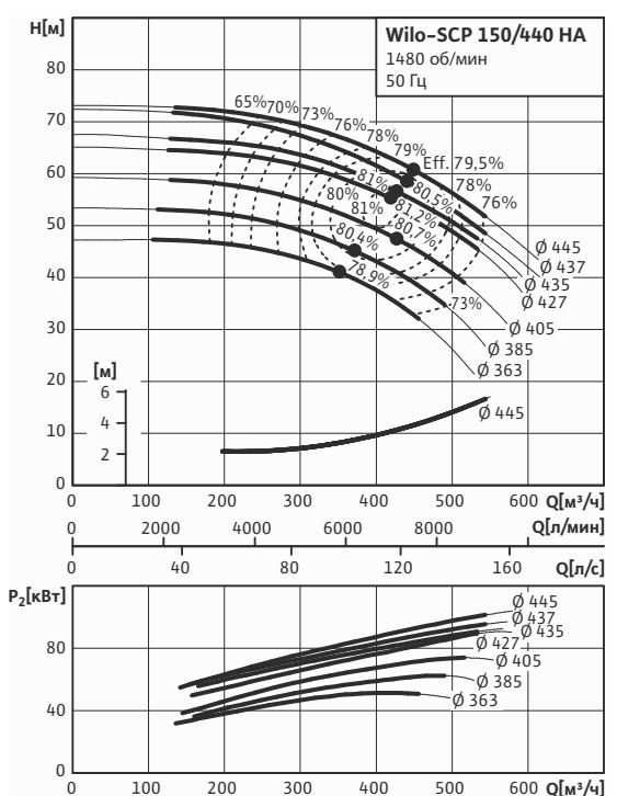
Wilо-SCP 150/440 HA
