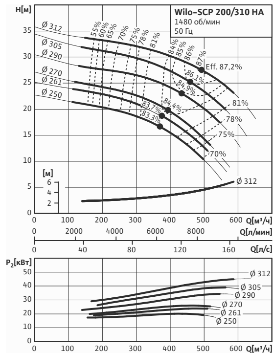
Wilo-SCP 200/310 HA
