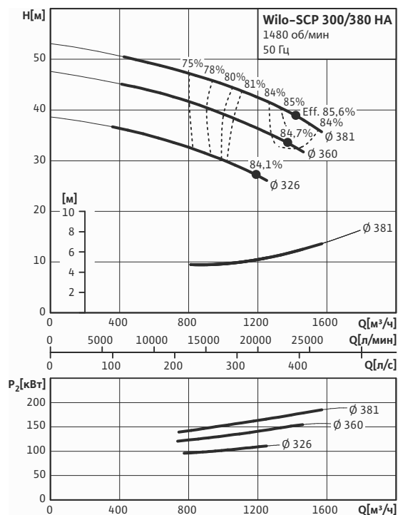
Wilo-SCP 300/380 HA
